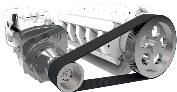
Riementrieb mit Planox®-Schaltkupplung
