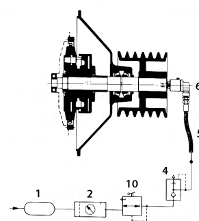
图13气动驱动a Planox®-离合器, PP型, 用于变量接合时的扭矩
